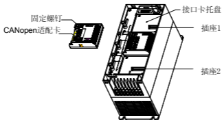
图 2 IOA-B105 通讯适配卡的拆卸安装示意图
