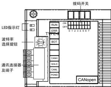
图 1 IOA-B105 适配卡的外观结构图
