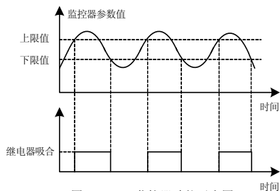
图 7-30-B 监控器功能示意图 2
