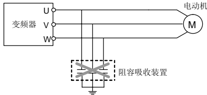
图 4-1 输出端禁止连接阻容吸收装置示意图
