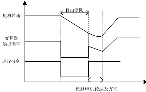
图 7-13 转速跟踪启动示意图
