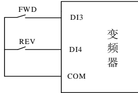
图 7-10-A 二线式运行模式 1
