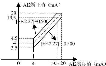
图 7-61-A AI2 零偏矫正曲线
