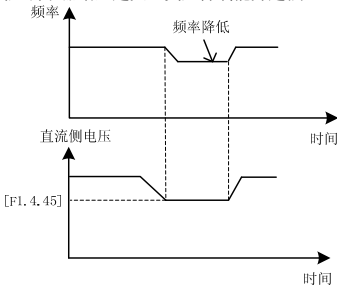
图 7-28-A 欠压调节示意图
