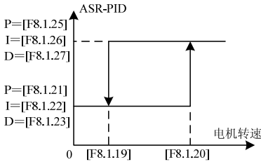
图 7-58-A 双 PID 参数（滞环切换）
