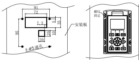
图 3-8-B 操作面板安装尺寸 2
