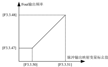
图 7-31 脉冲输出 Fout 特性曲线
