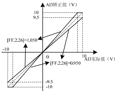
图 7-62-B-AI3 增益矫正曲线
