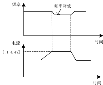
图 7-28-B 限流调节示意图
