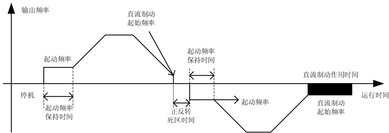
图 7-17 停机直流制动示意图
