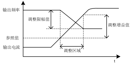
图 7-42 动平衡变量设置示意图
