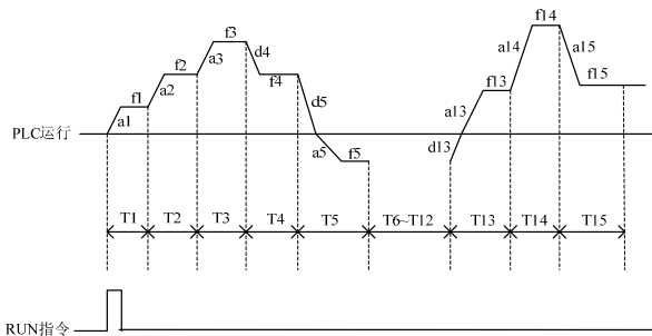
图 7-43-E 简易 PLC 运行保持最终值模式
