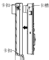
图 3-5 操作面板安装示意图
