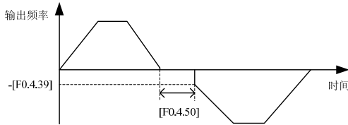
图 7-19 启动频率正反切换示意图
