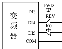
图 7-11-B 三线式运行模式 2
