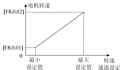
图 7-56 转速设定值和电机转速对应关系图
