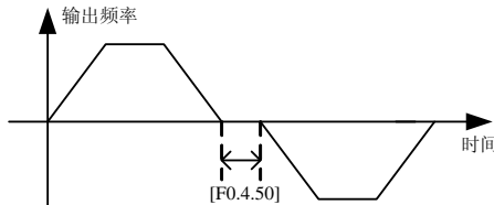
图 7-18 正反转过渡死区示意图
