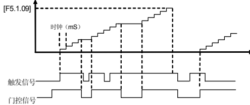
图 7-37-C
