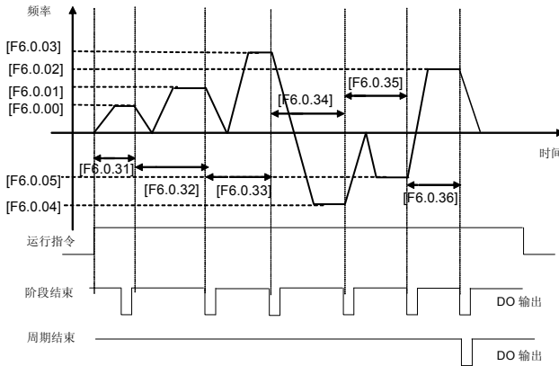
图 7-43-C 简易 PLC 运行单循环停机模式
