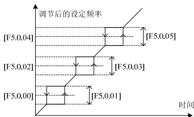
图 7-36 跳跃频率输出示意图
