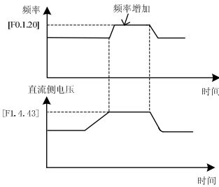
图 7-27-A 稳定运行过程的过压抑制
