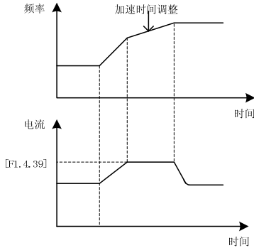
图 7-26 加/减速电流限制示意图
