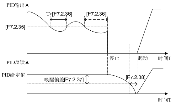
图 7-54 PID 睡眠功能示意图
