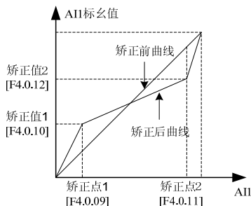
图 7-34 模拟输入 AI1 曲线
