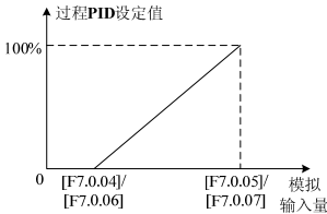
图 7-47 过程 PID 设定值定义示意图
