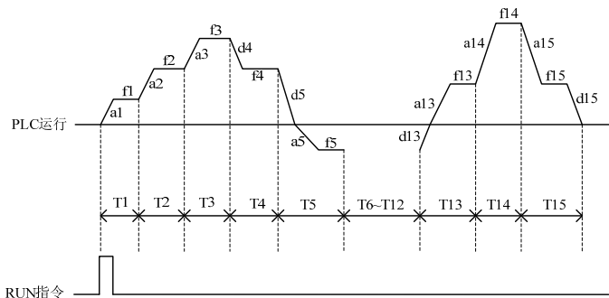
图 7-43-B 简易 PLC 运行单循环模式
