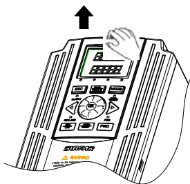
图 3-4 操作面板拆卸示意图
