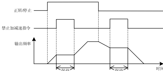
图 7-29 禁止加减速示意图
