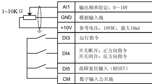
图 7-2-B 两线控制二 AI1 设定接线图
