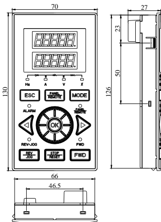
图 3-8-A 操作面板安装尺寸 1
