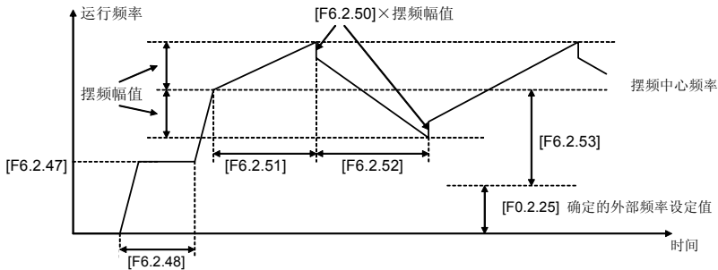
图 7-45 摆频运行示意图
