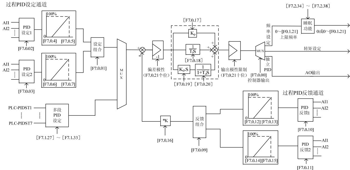
图 7-46 过程 PID 控制原理框图
