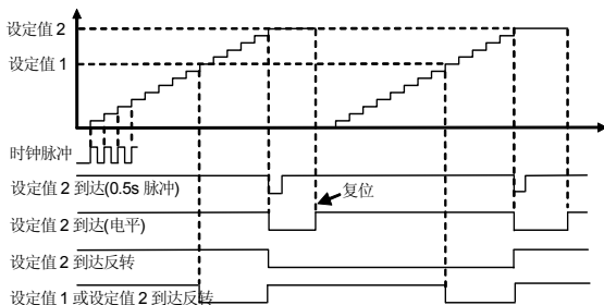
图 7-38-B 计数器功能 2
