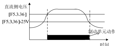
图 7-40 能耗制动
