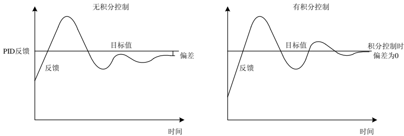
图 7-49 积分控制的作用
