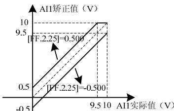
图 7-60-A AI1 零偏矫正曲线
