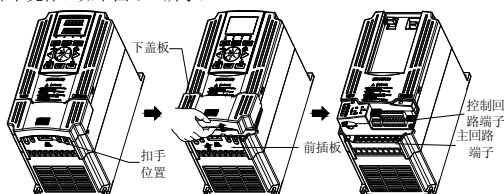
图 3-7 塑壳盖板的拆卸安装示意图
