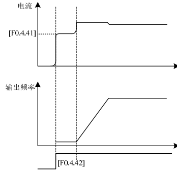
图 7-15 启动预励磁输出
