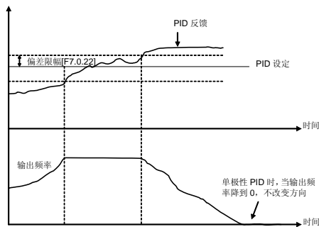
图 7-50-A 单极性 PID 控制方式
