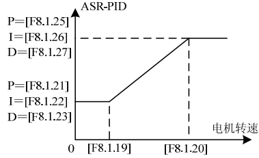
图 7-58-B 双 PID 参数（连续切换）
