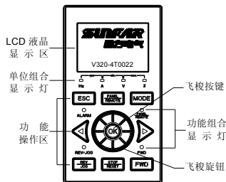
图 12-1 LCD 飞梭型
