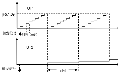
图 7-37-D
