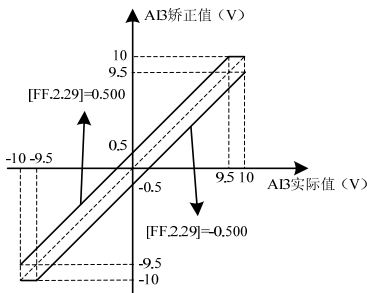
图 7-62-A-AI3 零偏矫正曲线
