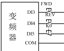
图 7-11-A 三线式运行模式 1
