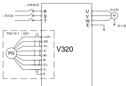
图 5-4 VC 运行接线图
