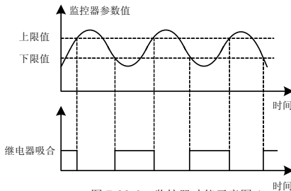
图 7-30-A 监控器功能示意图 1
