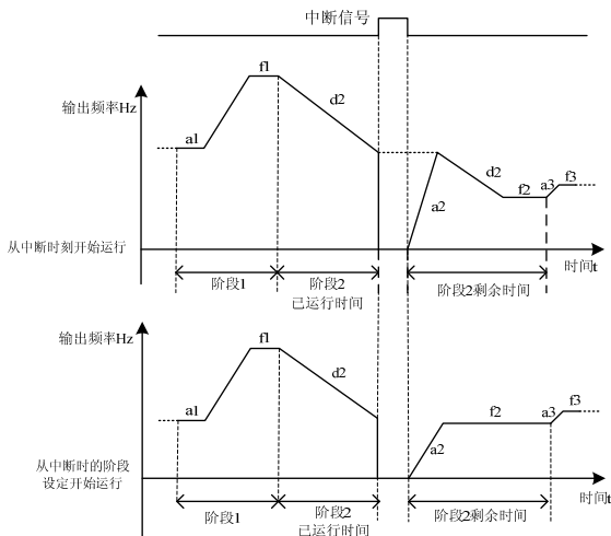
图 7-44 断点恢复示意图
