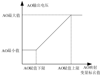
图 7-35 AO 输出特性曲线
