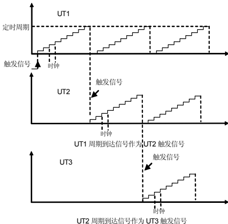
图 7-37-E 定时器 (UT1、UT2、UT3) 的触发串接功能
