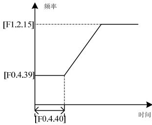
图 7-14 启动频率示意图
