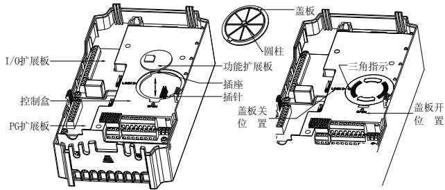
图 3-9 扩展板与功能板的安装拆卸示意图
