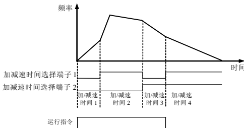
图 7-22 加、减速时间的外部端子选择方式
