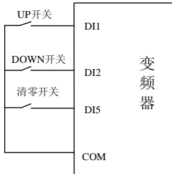
图 7-9 端子 UP/DW 接线示意图
