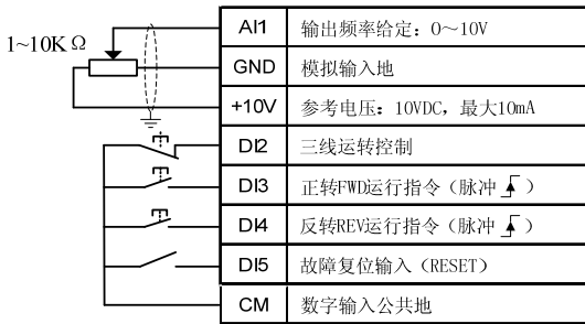
图 7-3 三线控制宏 AI1 设定接线图
