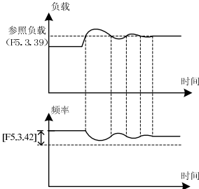
图 7-41 负载动平衡功能示意图
