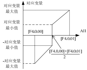
图 7-32-B
