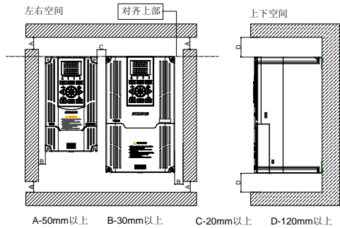
图 3-2 两台变频器（3.7KW 以上）左右安装尺寸
