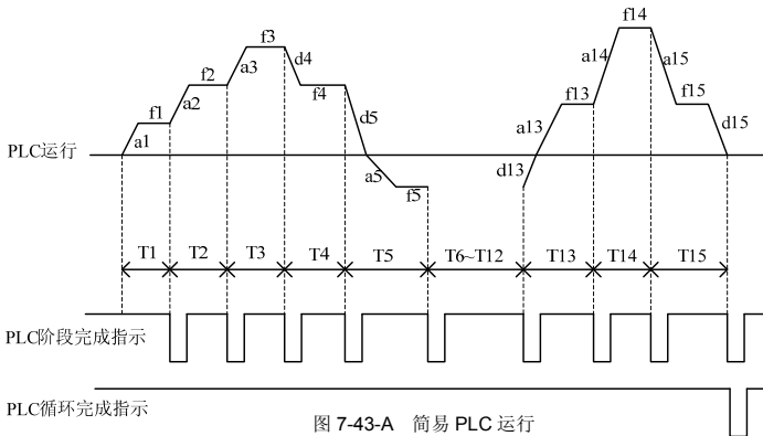
图 7-43-A 简易 PLC 运行
