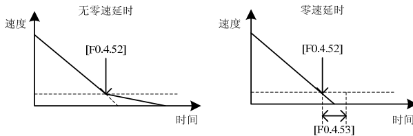
图 7-20 有无零速延时对比图
