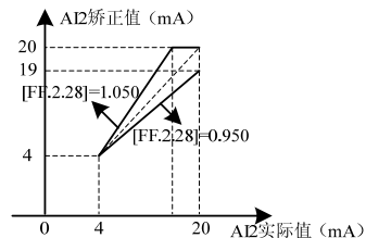
图 7-61-B AI2 增益矫正曲线
