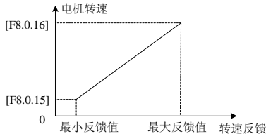
图 7-57 转速反馈值和电机转速对应关系图
