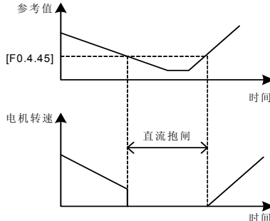
图 7-16 直流抱闸示意图
