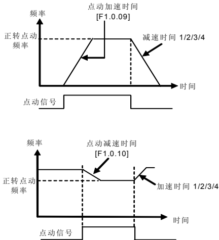
图 7-8 正转点动运行曲线
