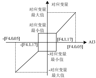
图 7-33-B
