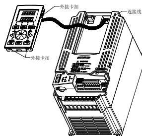
图 3-6 外延键盘连接图
