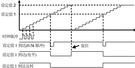
图 7-38-A 计数器功能 1
