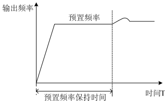
图 7-52 闭环预置频率运行示意图
