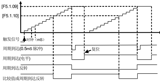
图 7-37-B
