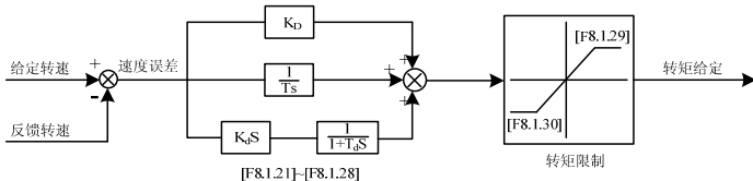
图 7-55 转速闭环框图
