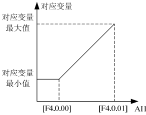
图 7-32-A
