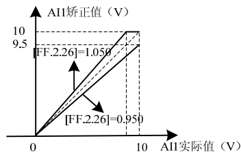
图 7-60-B AI1 增益矫正曲线
