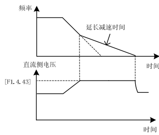
图 7-27-B 减速过程的过压抑制
