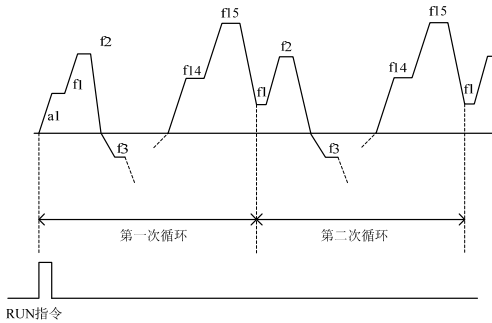
图 7-43-D 简易 PLC 运行连续循环模式
