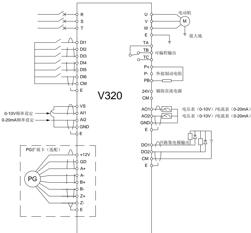
图 4-2 V320 系列变频器基本接线图
