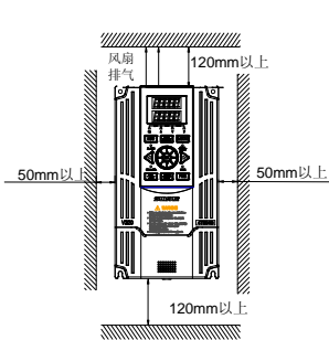
图 3-1 安装间隔距离
