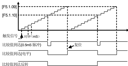
图 7-37-A
