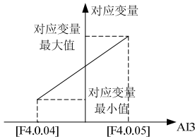
图 7-33-A
