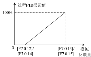
图 7-48 过程 PID 反馈值对应关系示意图
