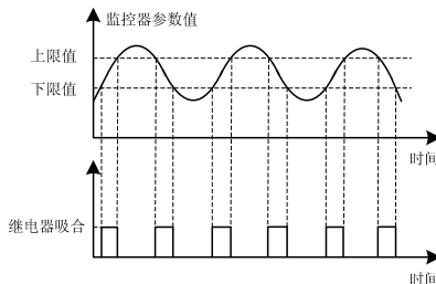
图 7-30-C 监控器功能示意图 3
