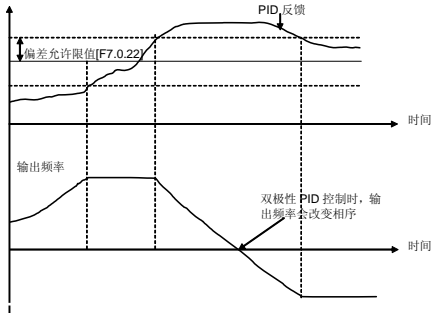
图 7-50-B 双极性 PID 控制方式
