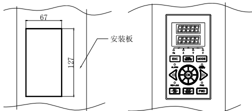
图 3-8-C 操作面板安装尺寸 3
