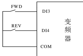
图 7-10-B 二线式运行模式 2
