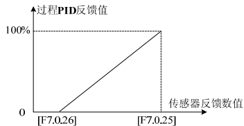
图 7-53 反馈百分比与对应传感器数值的关系曲线
