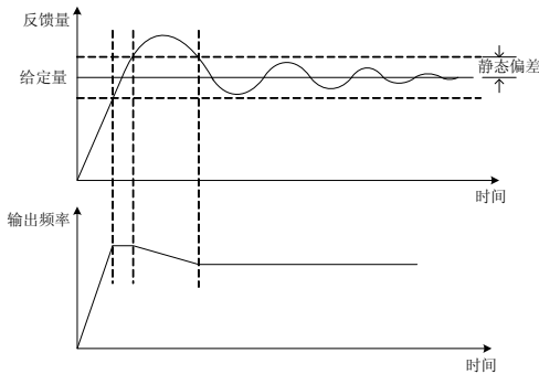
图 7-51 静态偏差示意图
