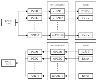
图5 PZD 数据通道示意图
