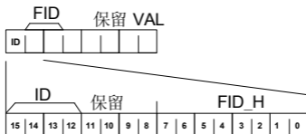
图 4 IOV-E108 适配卡通信报文 PKW 格式
