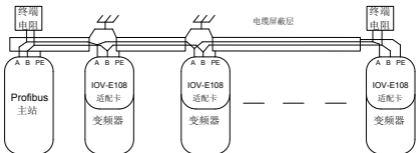
图 7 DP 通信适配卡安装图
