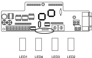
图 8 LED 指示灯图示
