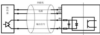
图 11 长线差分输出
