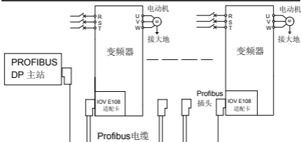
图 6 变频器与 Profibus 组网接线图
