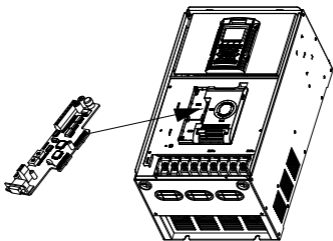
图 2 IOV-E108 适配卡的拆卸安装图
