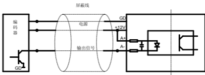
图 10 集电极开路输出
